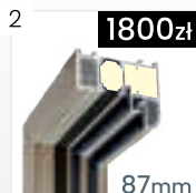
2 Ościeżnica aluminiowa ALU/90 trzykomorowa z podwójnym uszczelnieniem z przegrodą PCW wypełnioną pianą 87mm
