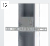
12 Elementy wzmacniające konstrukcję ościeżnicy z kotwami montażowymi Ościeżnica 15/54
